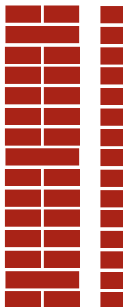
а) колодцева кладка
